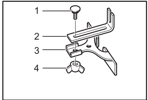
► 1. Bolt 2. Guide plate 3. Straight guide 4. Wing nut
