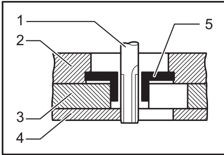
► 1. Bit 2. Base 3. Templet 4. Workpiece 5. Templet guide
