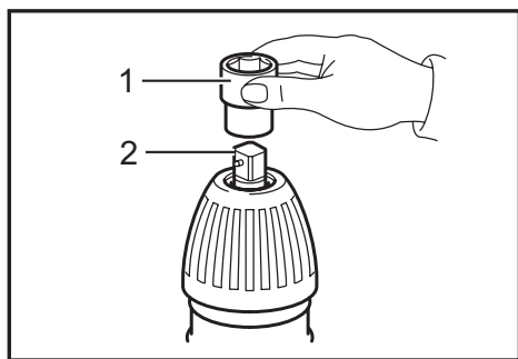
► 1. Socket 2. Anvil
