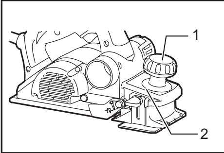
► 1. Knob 2. Pointer
